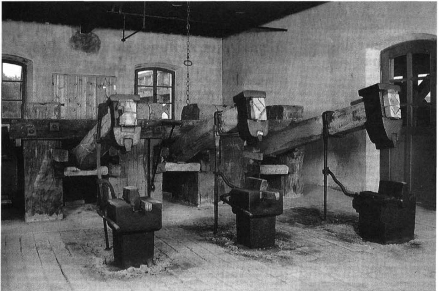
Durch ein unterschlächtiges Wasserrad angetriebenes Hammerwerk.
